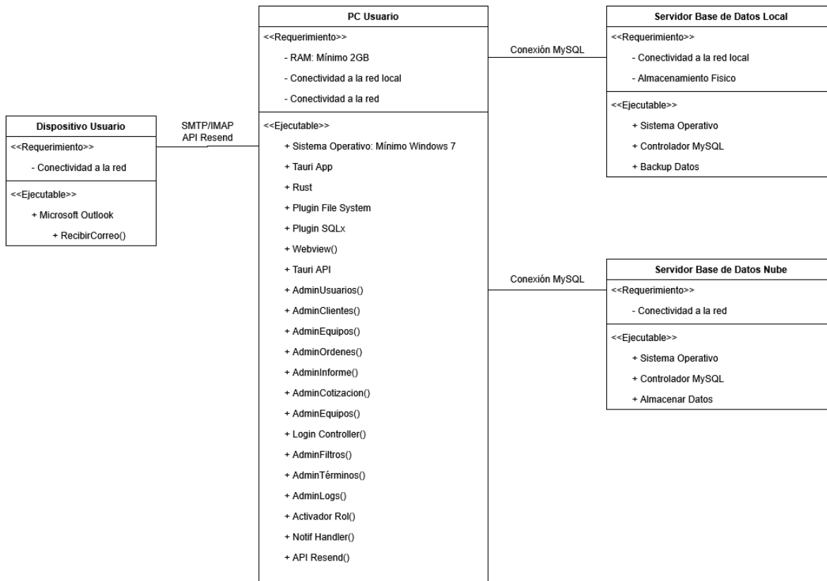
Figura 3.18 Diagrama de Despliegue del Sistema
