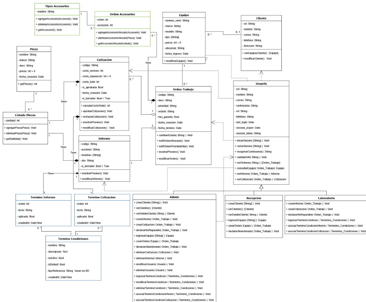
Figura 3.2 Diagrama de Clases de las entidades del sistema
