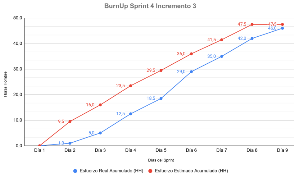
Figura 3.252 Gráfica BurnUp del esfuerzo de equipo en el Incremento 3
