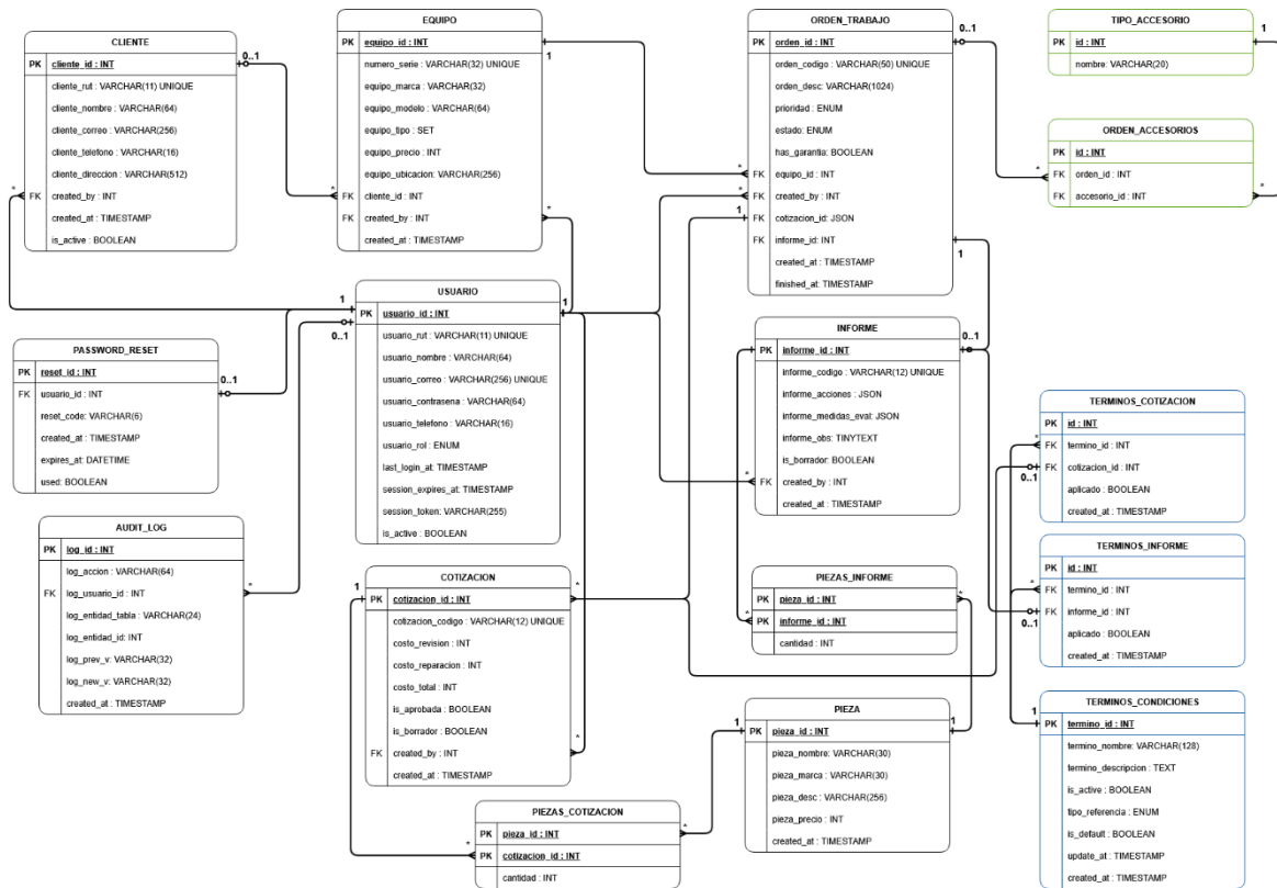
Figura 3.1 Modelo de base de datos del sistema
